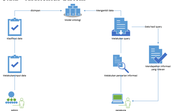
Gambar 6. Arsitektur sistem
