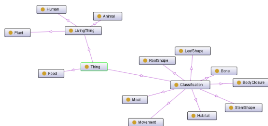
Gambar 8. Graph Ontologi kelas.
