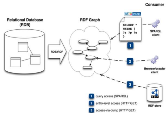
Gambar 4. Gambaran umum SPARQL (Prud'hommeaux dan Hausenblas, 2010.)
