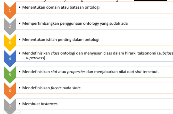
Gambar 7. Tahapan membangun ontology.
